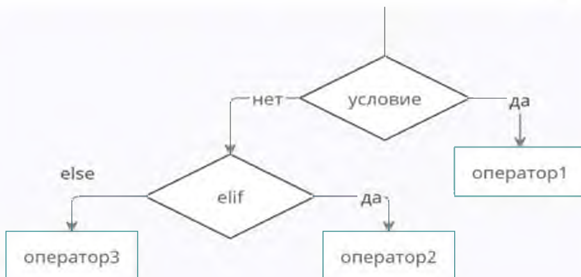
Рис. 51. Блок-схема условного оператора
