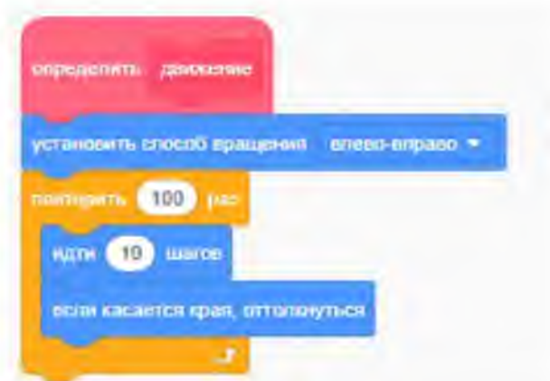
Рис. 146. Вид скрипта для нового блока
