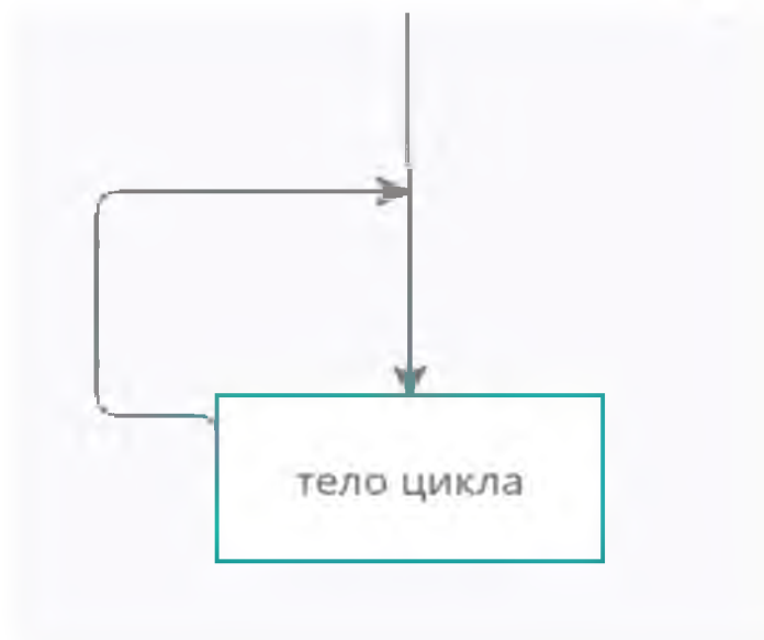
Рис. 126. Блок-схема цикла
