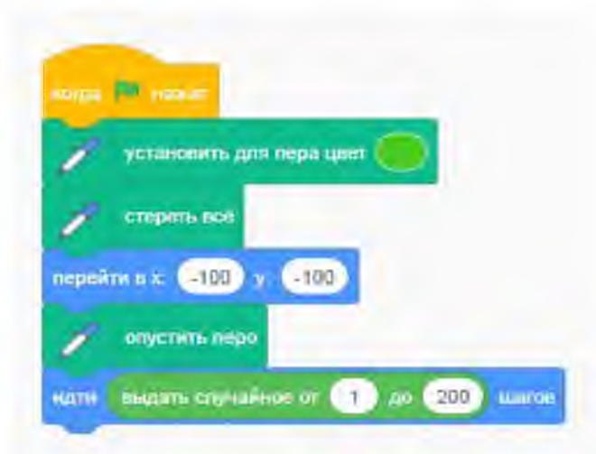
Рис. 106. Вид скрипта
