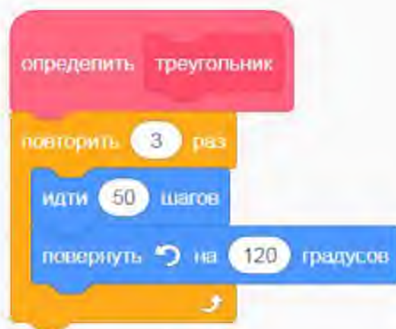
Рис. 136. Вид скрипта
