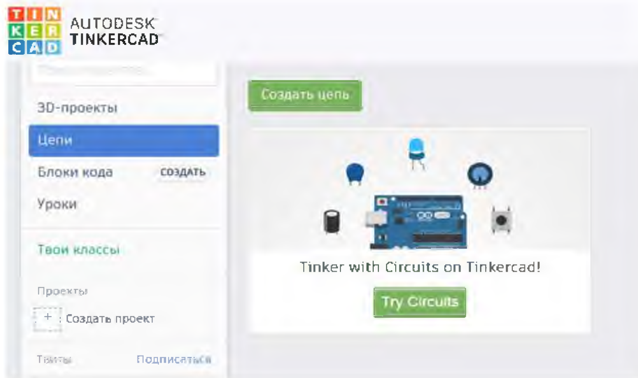
Рис. 161. Вид программы
