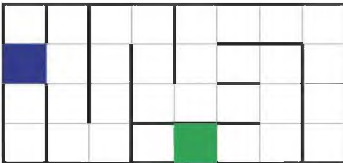
Рис. 2. Вид лабиринта
