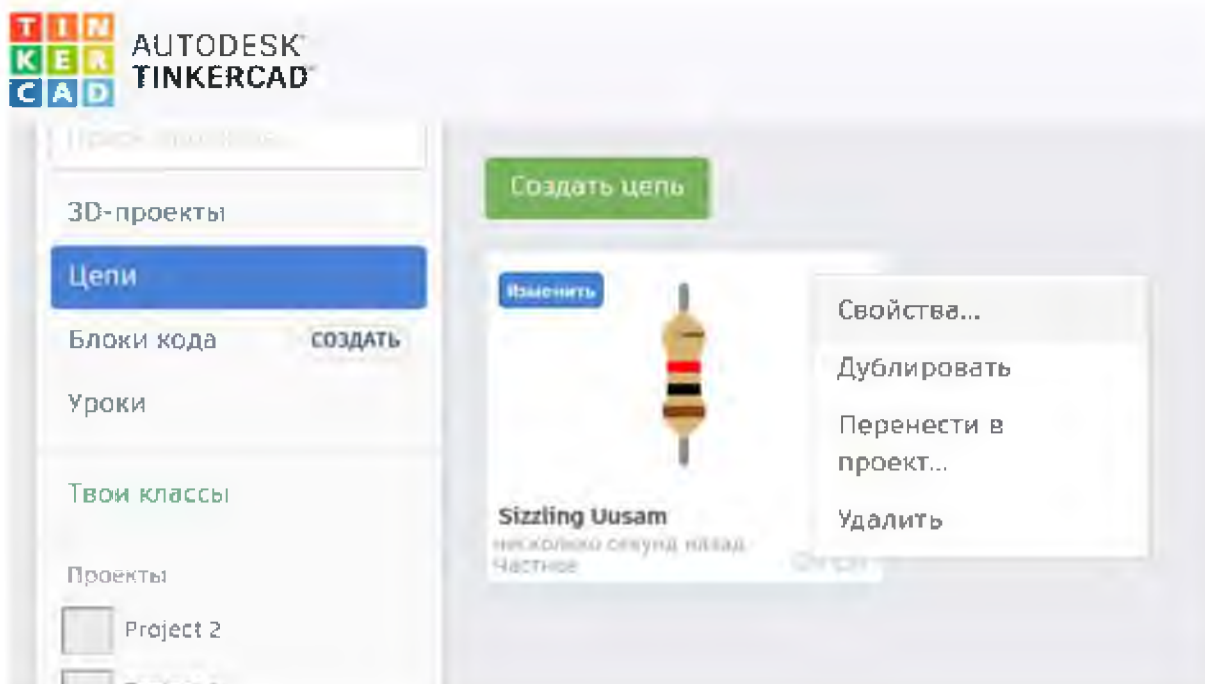
Рис. 162. Вид программы
