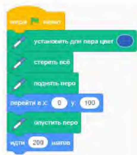
Рис. 103. Вид скрипта
