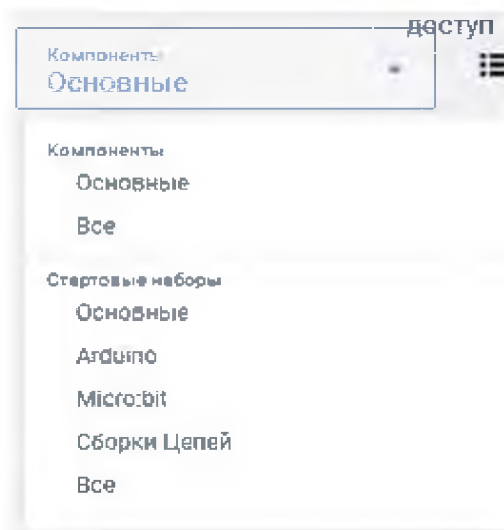
Рис. 168. Вид программы
