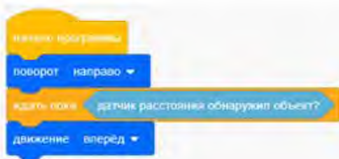
Рис. 32. Блок Ждать пока
