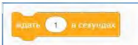
Рис. 17. Блок Ожидания
