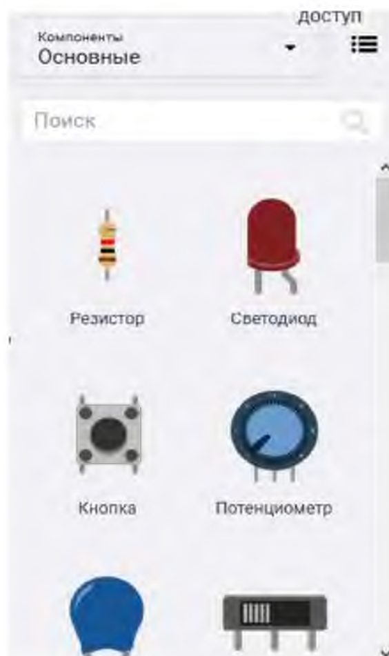
Рис. 167. Вид программы
