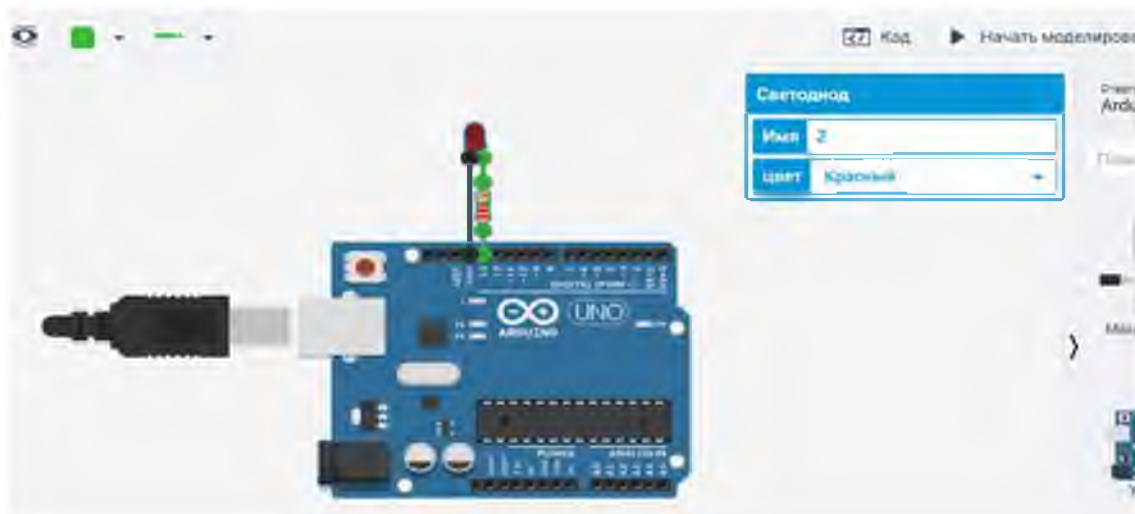
Рис. 170. Вид программы
