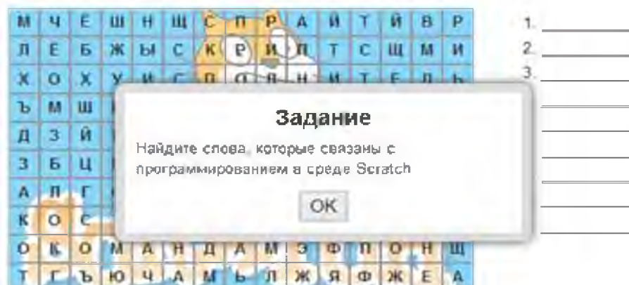
Рис. 174. Вид задания
