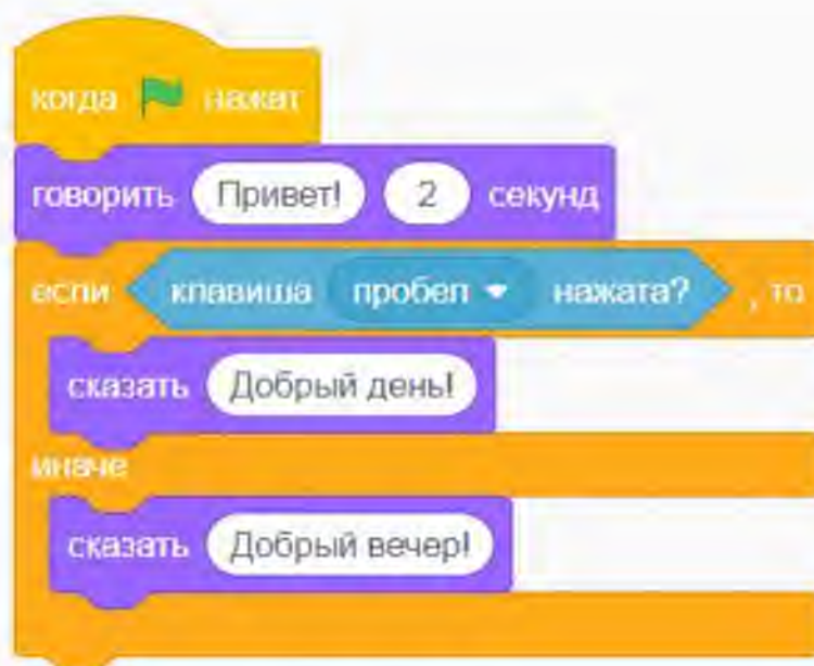
Рис. 122. Вид программы
