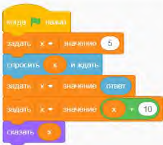
Рис. 117. Вид программы
