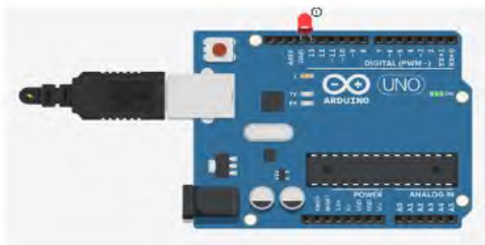
Рис. 166. Вид программы
