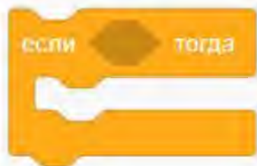
Рис. 21. Блок Если-тогда
